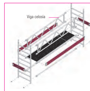
2c. Vigas celosía.
