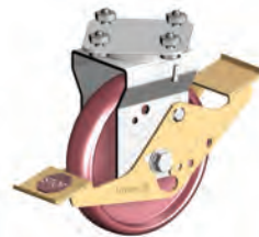
► Conjunto rueda 700 sin base regulable
