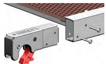
► Garra roja con remaches para plataforma
